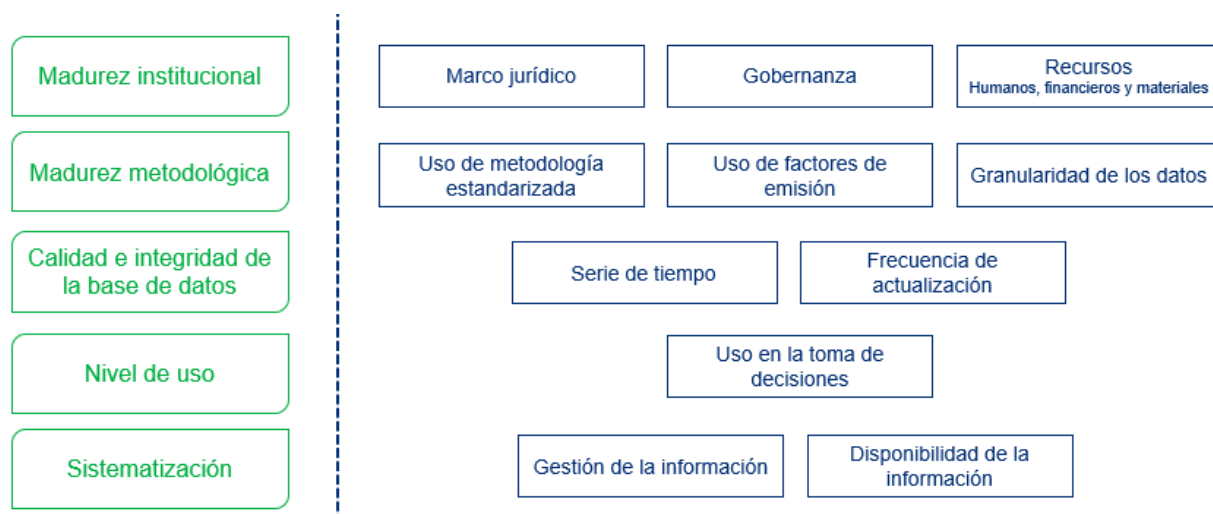
Figura 3.b Parámetros de evaluación definidos por criterio de madurez
