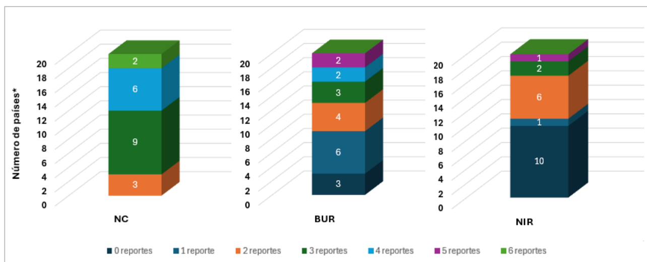
Figura 9. Número de reportes presentados a la CMNUCC por tipo y cantidad de países
