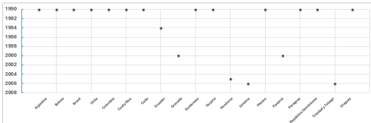
Figura 14. Fechas de inicio de las series históricas de los inventarios nacionales de GEI
