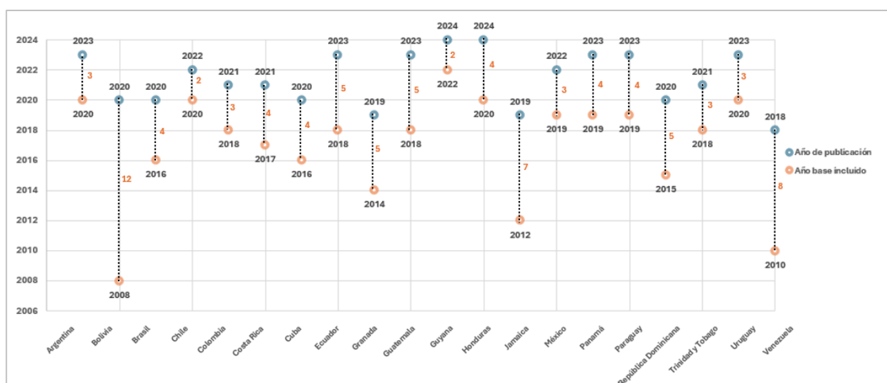
Figura 10. Márgenes temporales de publicación y año base de inventario más reciente
