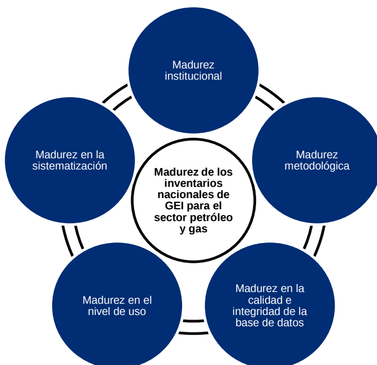
Figura 3.a Criterios de madurez definidos para evaluar los Inventarios Nacionales de GEI
