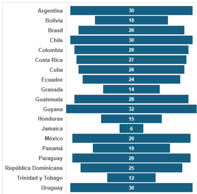
Figura 13. Rangos de las series históricas abarcadas en los inventarios nacionales de GEI
